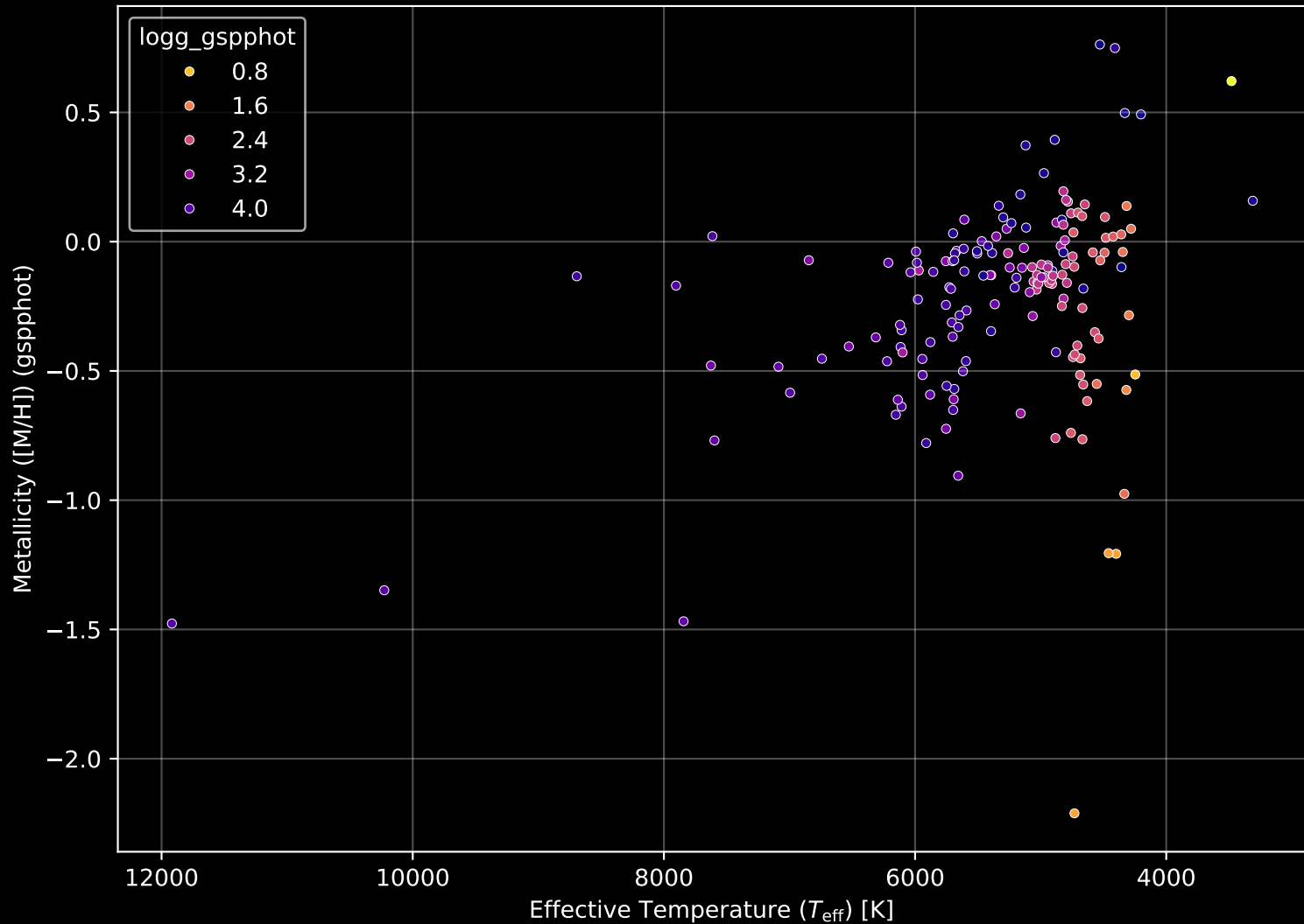
APOGEE DR17 Field: [269-22-O_TESS] Stellar Population Parameters (n= 165)
